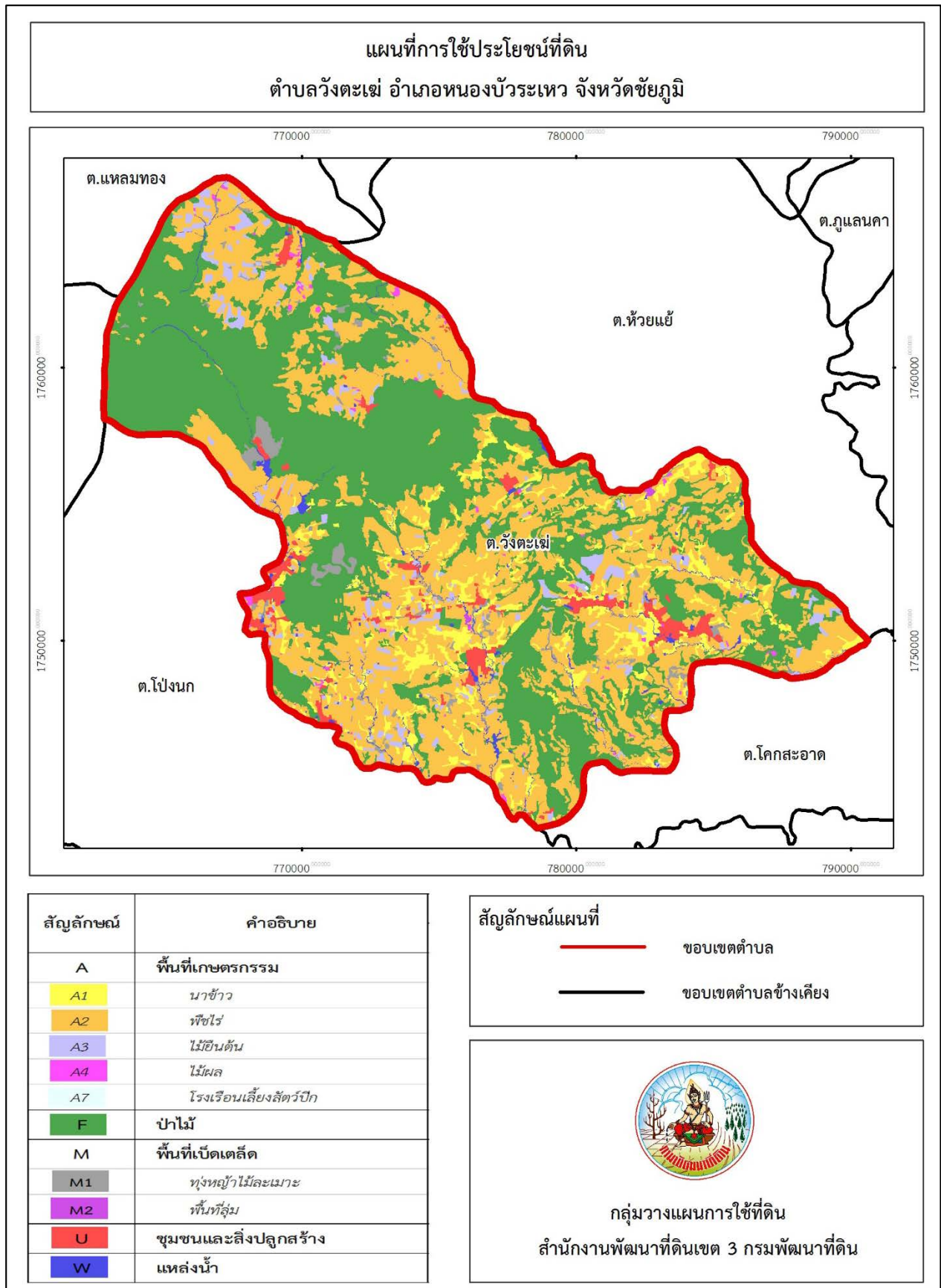
รูปที่ 2-4 สภาพการใช้ที่ดินตำบลวังตะเฆ่ อำเภอนองบัวระเหว จังหวัดชัยภูมิ
