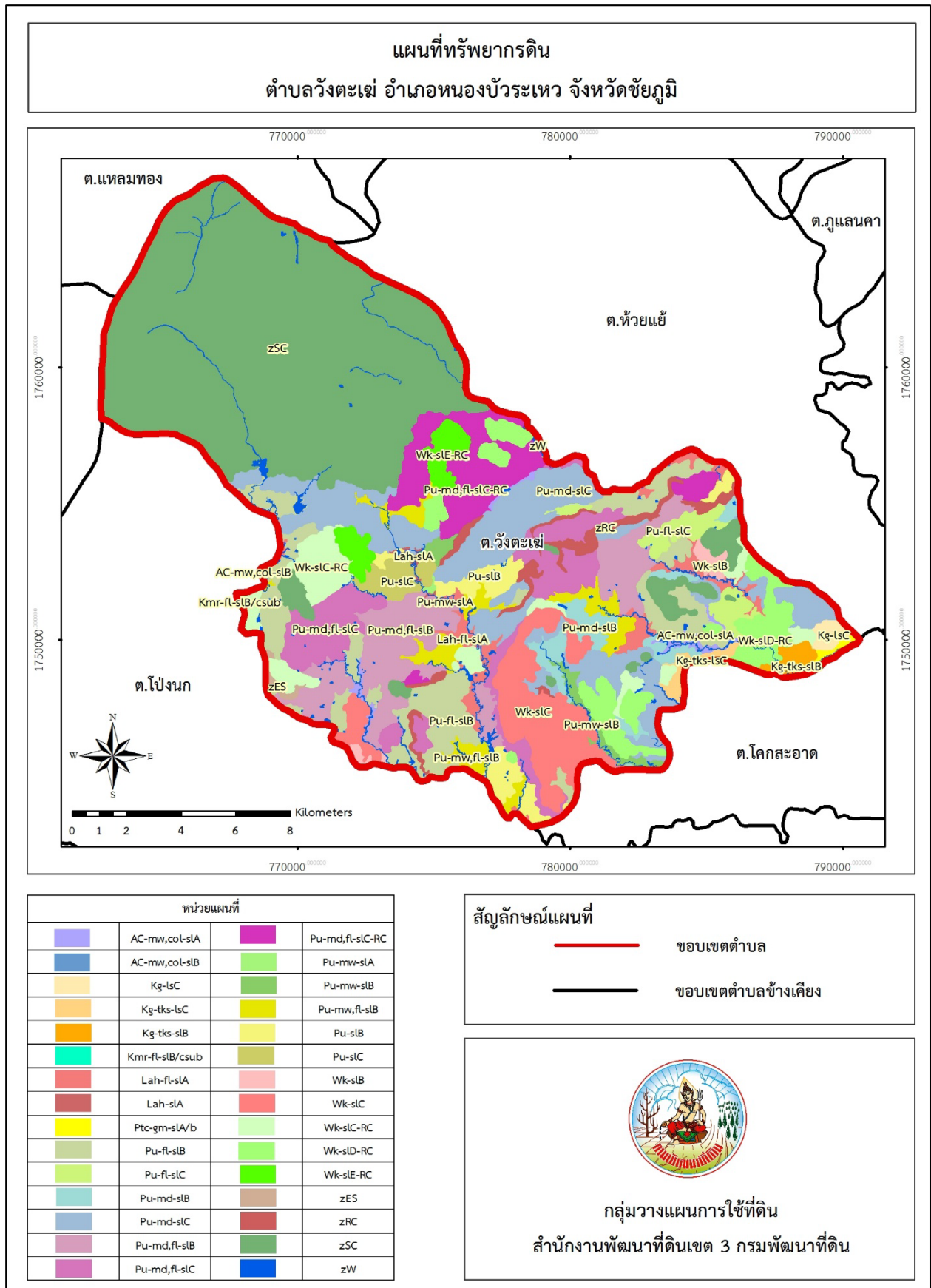
รูปที่ 3.4 ทรัพยากรดินตำบลวังตะเฒ่า อำเภอนองบัวระเหว จังหวัดชัยภูมิ
